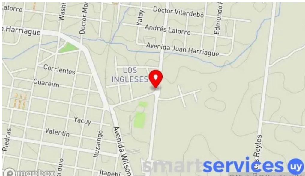
Gomeria 24h mapa
